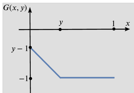
Σχήμα 3: Η γραφική παράσταση της G(x, y) που δίνεται από την σχέση (2.50).
