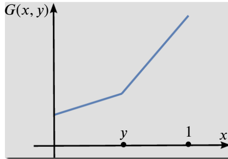
Σχήμα 2: Η γραφική παράσταση της G(x, y) που δίνεται από την σχέση (2.39).
