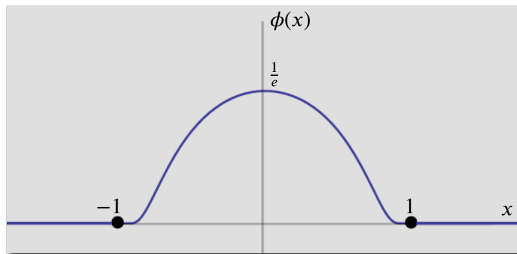
Σχήμα 1: Η γραφική παράσταση της \phi(x) που δίνεται από την σχέση (1.1)
