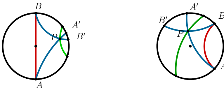
Σχήμα 9.3: Παράλληλες και υπερπαλλήλες \Delta -ευθείες της (AB) .
