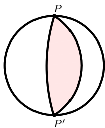
Σχήμα 5.1: 'τρακτος ή δίγωνο.
