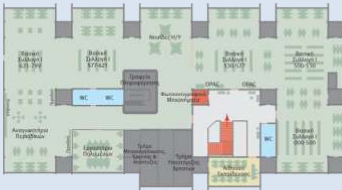
Κάτοψη δεύτερου ορόφου Β.Κ.Π.
